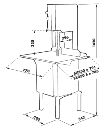
SX350 - SX350 S
